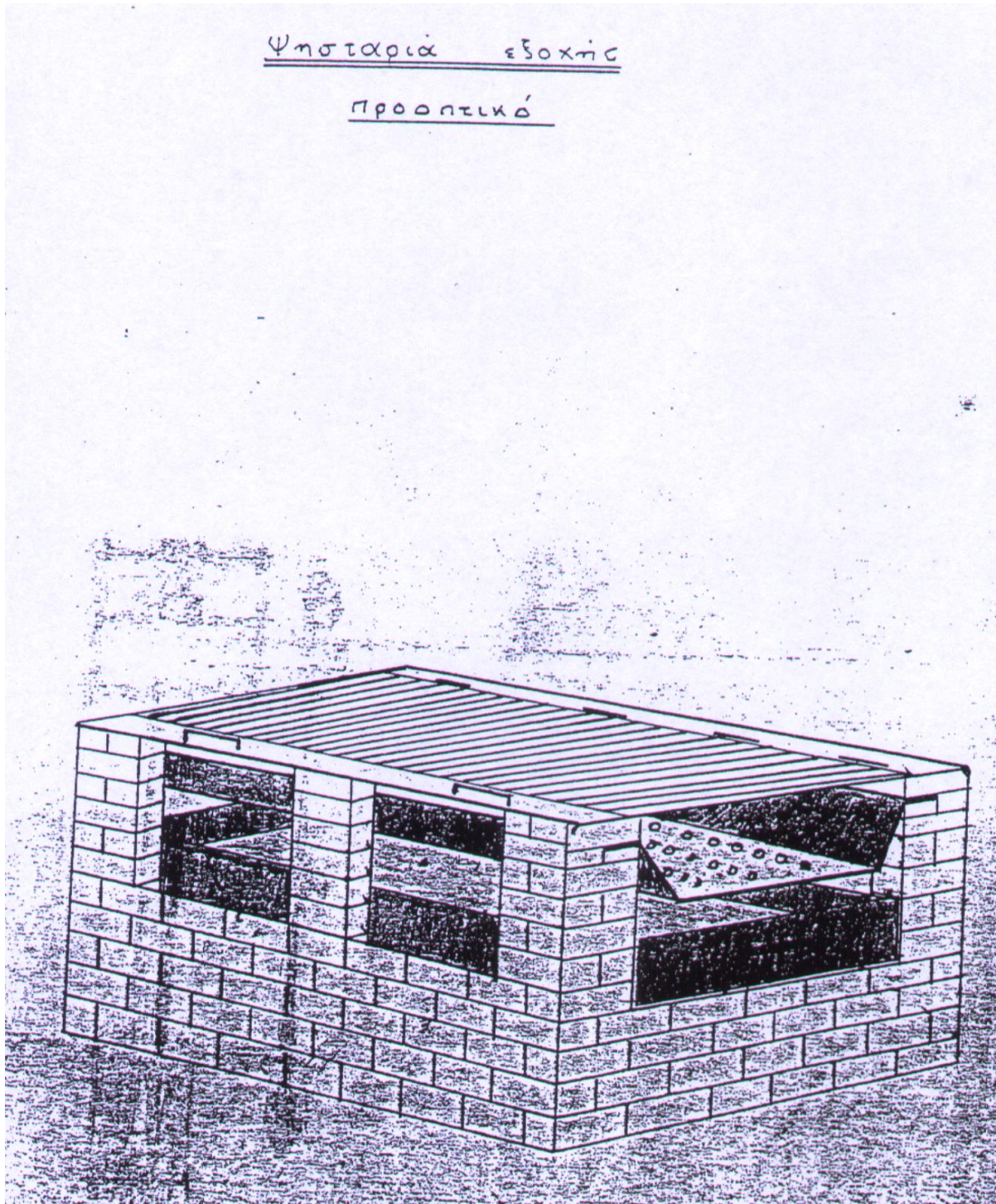
Σχέδιο 8 : Ψησταριά
